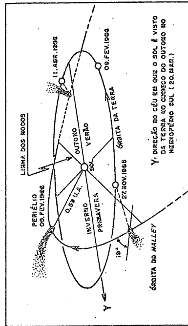
Trecho da órbita do Halley
